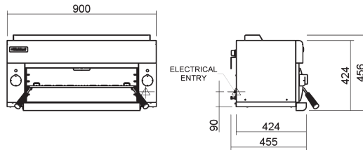
SN8200E
