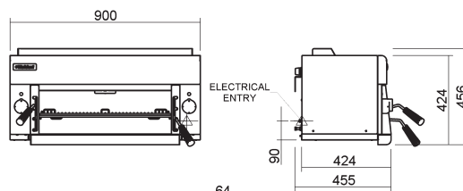
SN8200EA
